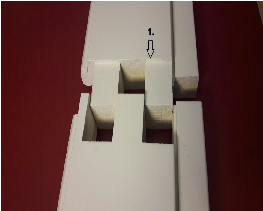
Kaski- ikkunakarmiliitos
